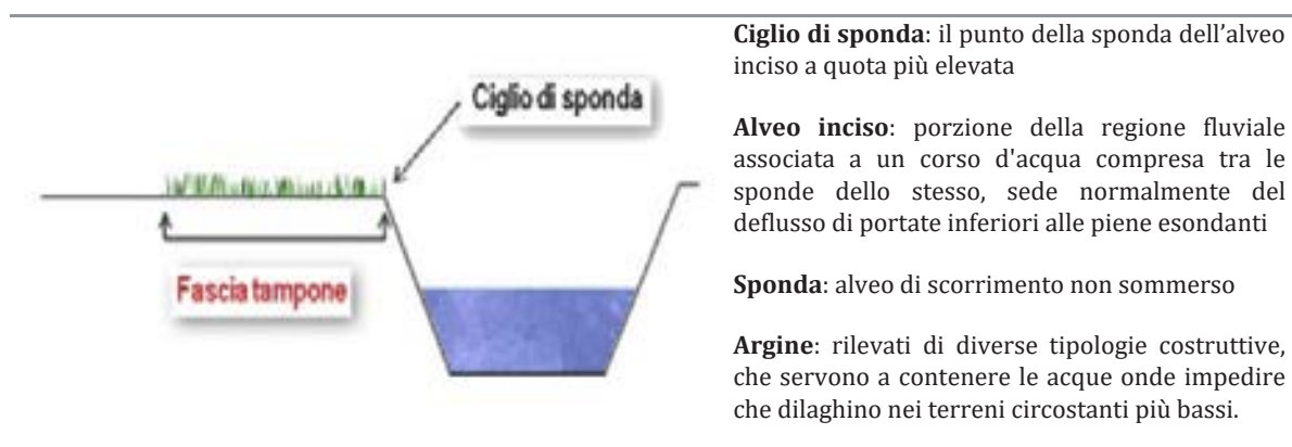
FIGURA 3: SCHEMA DI UN CORSO D'ACQUA CON FASCIA TAMPONE
